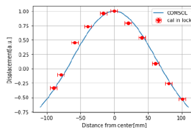
図 1: 形状が単純な 24kHz モードの形状の測定結果。横軸が鏡面の中心からの距離。縦軸が鏡面の変位。青線がシミュレーションの結果。赤がマイケルソン干渉計による測定値。再現性も確認された。
