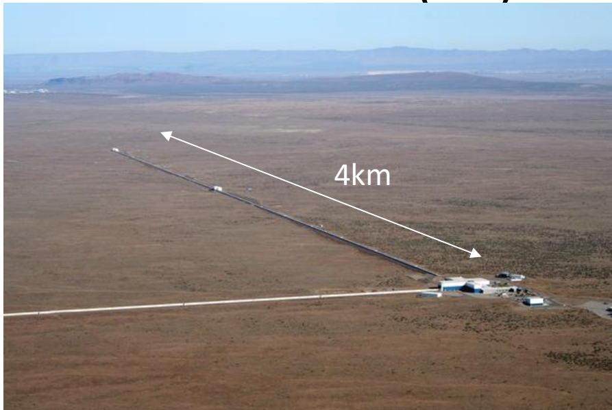
LIGO-Hanford(H1)
