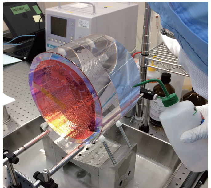
図5 直径 22 cm の無色透明のサファイアの鏡 A transparent sapphire mirror 22 cm in diameter
