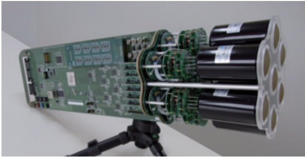
図4 日本グループが設計と製作を担当したカメラクラスターモジュール。7本の高量子効率光電子増倍管、高圧回路、プリアンプ、スロー制御回路、超高速DRS4波形読み出し回路、トリガーからなる。265個を集めて大口径望遠鏡のカメラになる。
