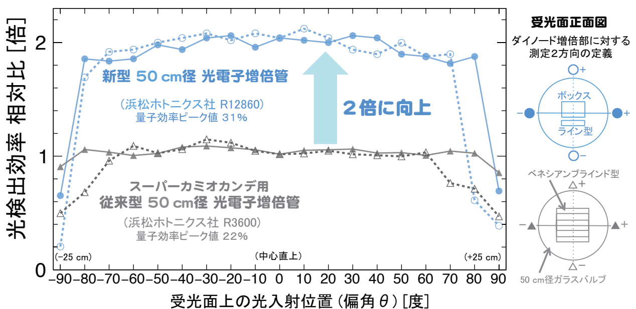
図2 現行 (黒) と新型 (青) 光検出器の検出効率の比較
