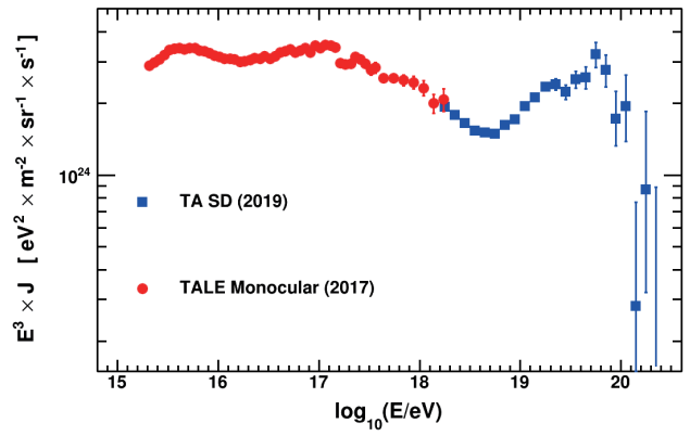
図3 TAの地表検出器 (■) とTALE望遠鏡 (●) で測定した超高エネルギー宇宙線のエネルギースペクトル。 Energy spectra of UHECRs measured with the TA surface detector (■) and the TALE telescope (●).
