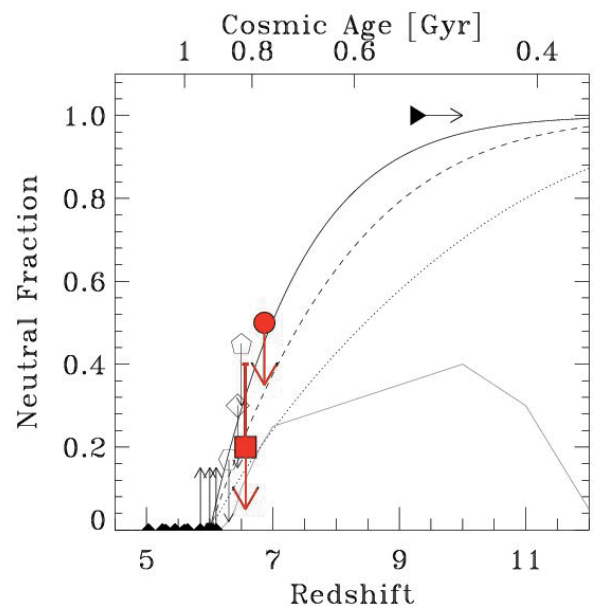
図5 これまでの研究で明らかにされた宇宙再電離の歴史。赤方偏移（横軸）に対する中性水素比（縦軸）の進化。赤印が Suprime-Cam の探査から付けられた制限。4つの曲線は異なる理論モデル。いつ、どのように宇宙再電離が進んできたかはほとんど分かっていない。 History of cosmic reionization, so far, understood. Red symbols denote constraints from our Suprime-Cam survey. Four lines represent different theoretical predictions. The epoch and process of cosmic reionization are unknown.
