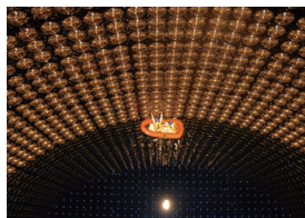
Super-Kamiokande
