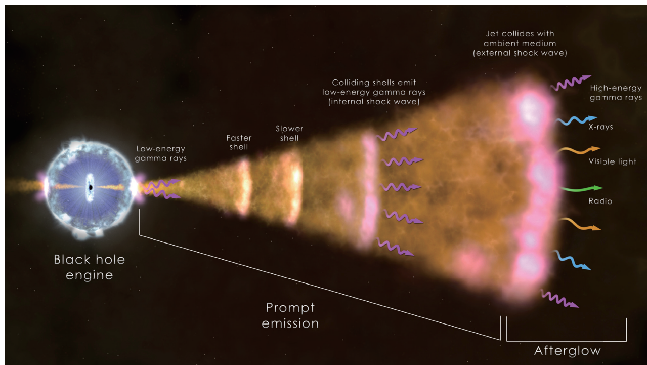
図2 ガンマ線バーストの想像図。巨星がその寿命に至り、中心核が重力崩壊を起こし、ブラックホールを形成する。そこへ星のガスが降着し、細く絞られた相対論的なジェットを放つ。ジェットは星表面を突き破り、星間空間へ飛び出す。そこで衝撃波を形成し、数十秒間に渡ってガンマ線を放ったり、徐々に暗くなる電波からX線での残光を放ったりする。©NASA's Goddard Space Flight Center
