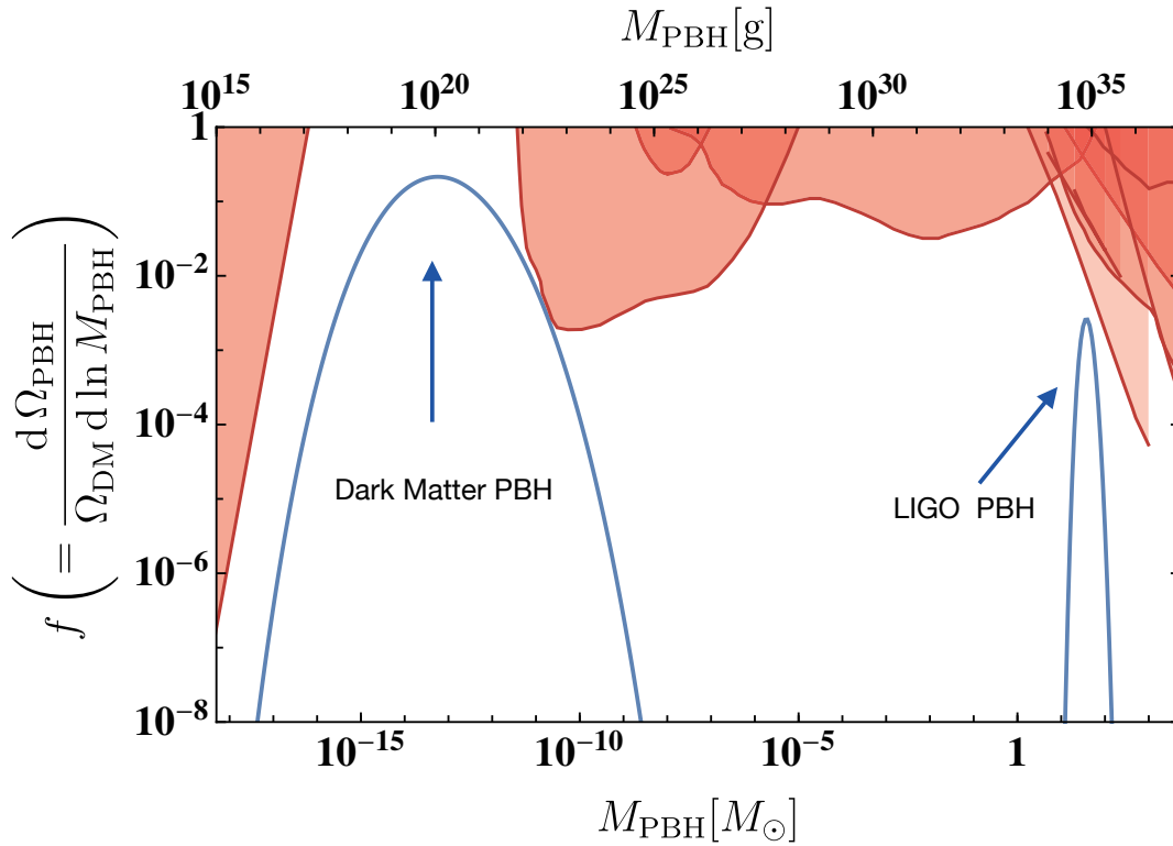
図1 ダブル・インフレーションで生成される原始ブラックホール（PBH）の質量分布。実線が理論的予言を表し、オレンジの領域が観測の制限を表す。質量の軽い PBH は宇宙の暗黒物質を説明し、質量が大きな PBH は重力波検出器 LIGO で見つかったイベントを説明できる。 Mass distribution of primordial black holes (PBHs). Solid curves represent the theoretical prediction and the orange shadows show the present observational constraints. Light PBHs can account for dark matter of the universe and heavy PBHs can explain the gravitational wave events discovered by LIGO.
