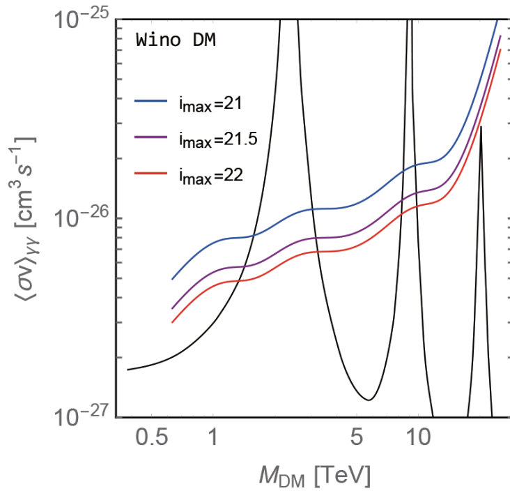
図2 ガンマ線に対消滅するウィーノ型暗黒物質に対する CTA 実験で期待される感度曲線。ここでは矮小楕円体銀河 Ursa Major II, Coma Berenices, Seque 1, Ursa Major I を 50 時間ずつ測定することを仮定。(黒：理論計算による対消滅断面積。青、紫、赤：矮小楕円体銀河からのガンマ線に対する CTA 実験感度。$i_{\text{max}}$ は暗黒物質密度測定に用いる矮小銀河星の上限等級) Sensitivity lines of CTA for Wino dark matter annihilating into two photons. Here, we assume 50 hours observation for the ultra-faint dwarf spheroidal galaxies, Ursa Major II, Coma Berenices, Seque 1, and Ursa Major I. (Black line: the predicted annihilation cross section. Colored lines : The sensitivity lines of CTA for given upper bounds on the member star magnitude used to estimate the dark matter density in the dwarf spheroidal galaxies.)
