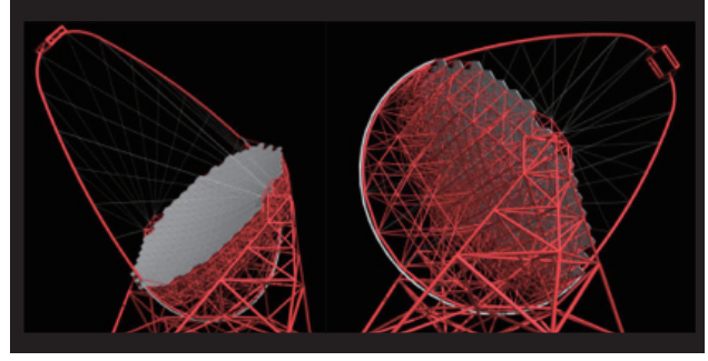
図3 大口径望遠鏡(23m口径)。日本グループは高分解能イメージングカメラ、超高速読み出し回路、高精度分割鏡のデザイン、光学補償装置の量産をすすめている。
