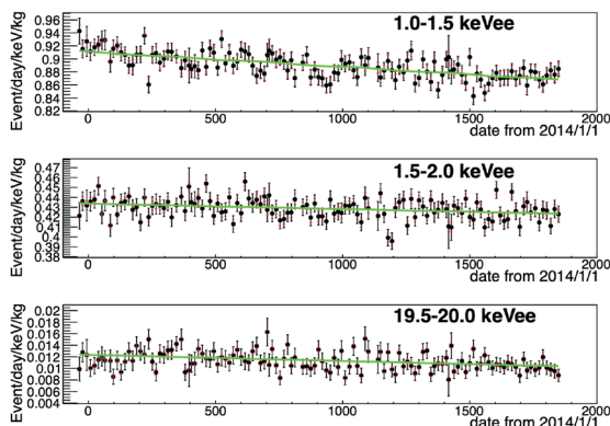
図5 観測されたデータの頻度を、エネルギー領域ごとに分けて時間推移を示したもの(黒点)。緑線は、暗黒物質が衝突している現象が含まれるとした場合に季節変動があるかどうか判定するために期待値でフィットしたもの。有意な振動は観測されなかった。
