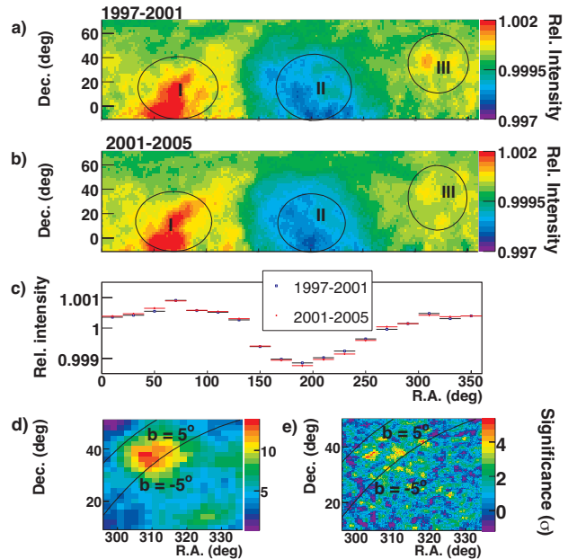
図6 シグナス領域 (III) のガンマ線点源探索 (e) の赤いホットスポットに注目) Search for gamma ray point sources in the Cygnus region ( III ). Watch out the hot red spots in e), please.
