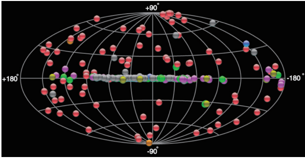
図2 超高エネルギーガンマ線源(>100GeV)を銀河座標系に示したもの。200以上の銀河内、銀河系のガンマ線源が発見されている(TeVCATカタログより引用)。
