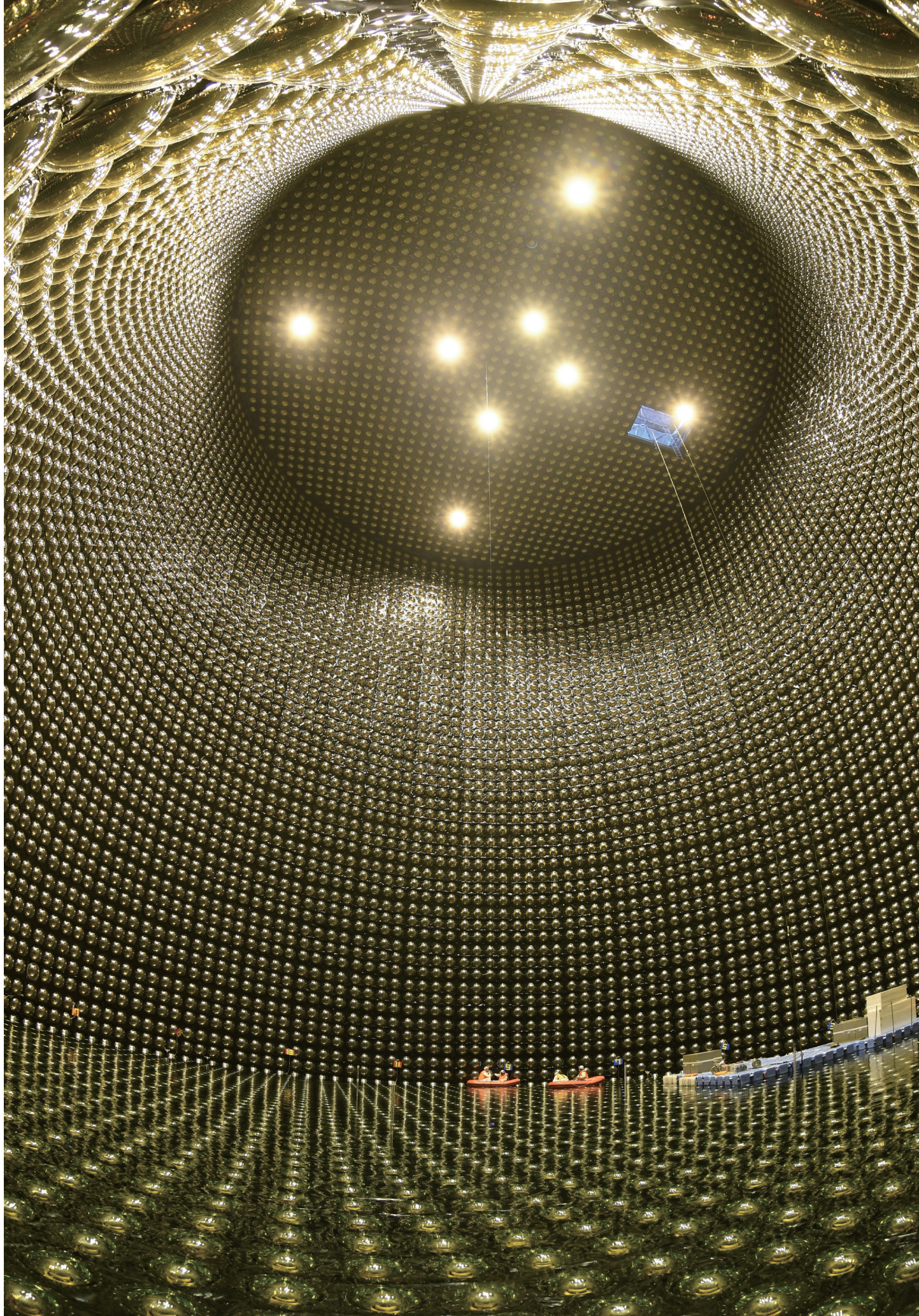
Super-Kamiokande
