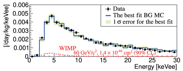
図4 検出器中心部で生じた事象の頻度。横軸は発光の強さを示す。黒い点はデータを示し、縦の棒は誤差を示す。青い線は見積もられたノイズの量で、緑のバンドはノイズ量の評価の誤差を示す。解析の結果、データはノイズと矛盾がなく、有意な暗黒物質の信号は観測されなかった。赤い点線は、得られたデータから考えられる暗黒物質の寄与の最大許容量を示す。
