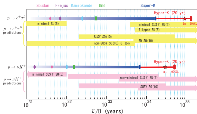
図4 核子崩壊の発見寿命感度（図中の赤い星印）と、スーパーカミオカンデ実験などによる下限値。バンドは大統一理論の予言範囲。横軸は、各崩壊モードでの核子寿命（核子寿命を分岐比 B で割ったもの）である。Hyper-K's discovery reaches for nucleon decays (red stars) compared with the experimental limits obtained by Super-K and other past experiments. Bands show predictions by various grand unified theories. X-axis shows nucleon lifetime divided by the branching ratio.
