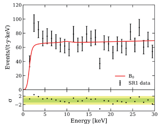
図6 XENON1T 実験の電子反跳現象のエネルギースペクトル。黒点がデータ、赤線がノイズの期待値を示す。2-4 keV 付近にノイズを超過したデータが見られる。
