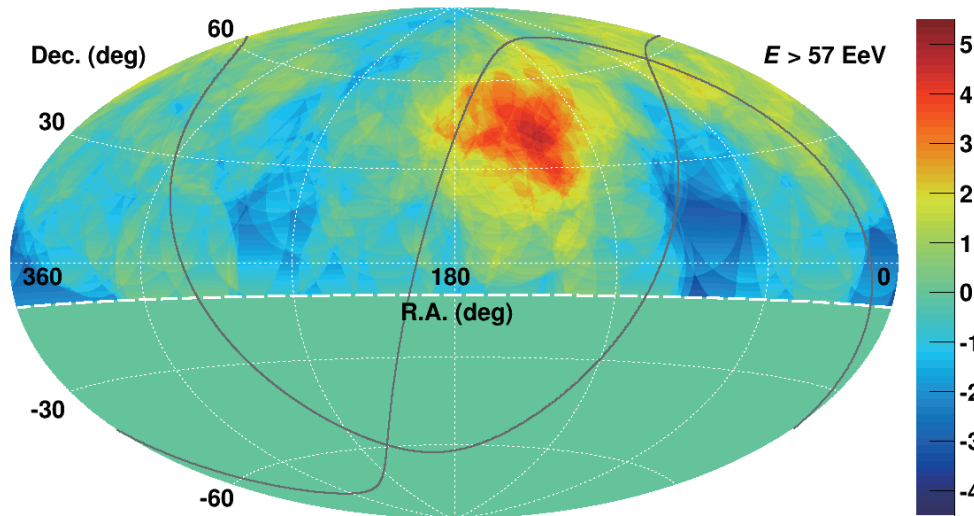
図5 TAで観測した 5.7 \times 10^{19} 電子ボルト以上の宇宙線の到来方向を半径 25^\circ の円でオーバーサンプリングした場合の統計的な有意度を示した天球マップ（赤道座標表示）。赤経 144.3^\circ 、赤緯 40.3^\circ を中心としたところに赤く有意度の高いホットスポットが見られる。 Hammer projection of the statistical significance of TA cosmic ray events with energies greater than 5.7 \times 10^{19} eV with 25^\circ -radius circle oversampling in the equatorial coordinates. The maximum excess appears as a hotspot centered at right ascension of 144.3^\circ and declination of 40.3^\circ .
