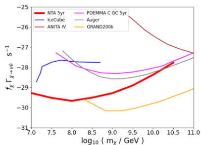
図5: 暗黒物質粒子 \nu_\tau 感度比較
