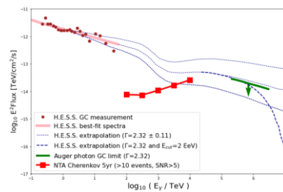
図6: 銀河中心 \gamma 線感度比較
