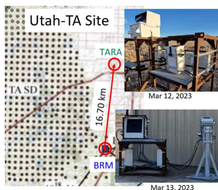
図1: ユタTAサイトの観測装置
