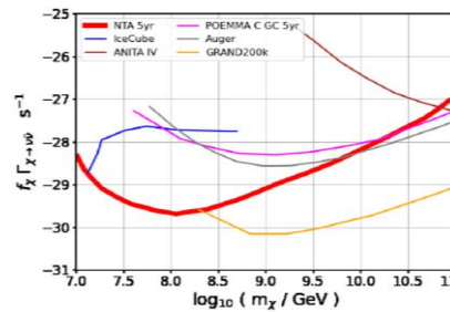
図5: 暗黒物質粒子 \nu_\tau 感度比較
