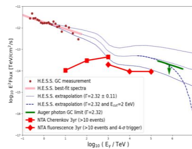
図6: 銀河中心 \gamma 線感度比較
