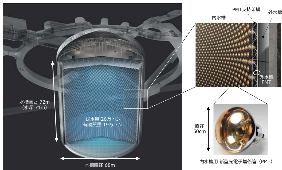
図 2 建設中のハイパーカミオカンデ装置の概念図
