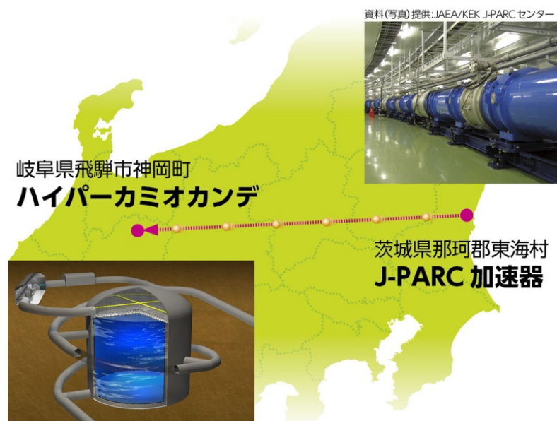
図 1：増強した J-PARC 加速器によりニュートリノビームを生成し、295km 離れた神岡町地下に建設されたハイパーカミオカンデで観測する。
