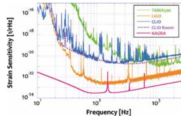
図2 KAGRAの感度曲線(赤線)とTAMA(緑線)、100メートルプロトタイプ低温干渉計CLIO(青線)の低温感度。紫の破線で示す室温究極感度が100Hz付近でわずかに上回っているのは低温鏡による低減効果を示している。なお、橙色の線で示したプロットは、現在最も感度が良いとされる米国の計画LIGO(基線長4km)で達成されている感度。
