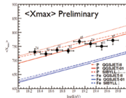
図4 TAで測定した超高エネルギー宇宙線の平均X max とエネルギーの関係。
