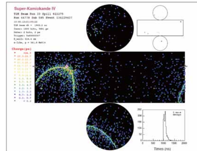
図1 スーパーカミオカンデで観測された、電子ニュートリノ反応候補事象の一つ。円筒形をしたスーパーカミオカンデの展開図で、内壁に配置された光電子増倍管の内、光を捉えたものにとらえた光の強度に応じて色をつけて表示している。水と電子型ニュートリノ反応によって発生した電子が引き起こす電子・陽電子シャワーが発生したチェレンコフ光がリング状に捉えられている。
