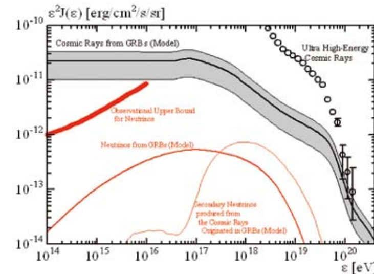
図2.ガンマ線バーストから放出される最高エネルギー宇宙線とニュートリノの見積りを示します。宇宙線の一部を説明しつつ、ニュートリノの観測的制限も避けられています。
