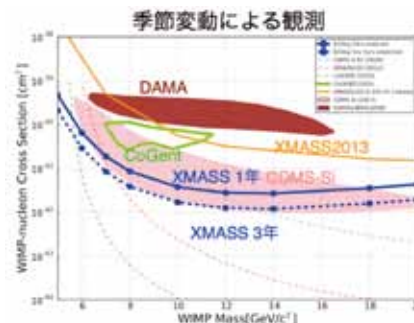
図6 改修後の観測で期待される季節変動を用いたXMASS実験による感度曲線(青線)。1年観測を続ければ季節変動を用いた暗黒物質探索において世界で最も感度があると予想されている。 Fig.6 Expected sensitivity for annual modulation by XMASS after refurbishment (blue line). XMASS will be the most sensitive detector for the dark matter annual modulation after 1 year data taking.
