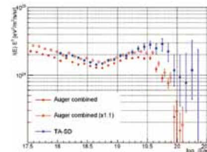
図3 TAの地表検出器(SD)で測定した超高エネルギー宇宙線のエネルギースペクトル(●)および南米アルゼンチンのAuger実験によるエネルギースペクトル(●)。○はエネルギーを10%大きくした場合のAugerのエネルギースペクトル。
