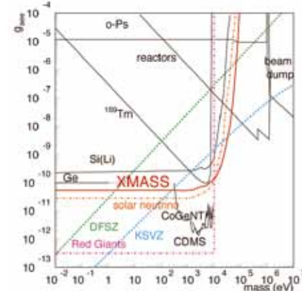
図4 結合定数 g_{ee} に対する制限曲線。実線は観測による制限で破線は理論で予想されるモデル、さらにRed Giantsおよびsolar neutrinoからの制限を表している。 Fig.4 Limit on the G ee coupling constant. Solid lines indicate the experimental limit and dashed lines for theoretical model that include Red Giants and solar neutrino constraints.
