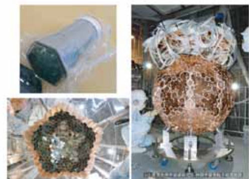
図2 XMASS実験用「極低放射能」光電子増倍管(Hamamatsu R10789)の据付作業の様子。642本の光電子増倍管の取り付け作業が完了。(右写真)
