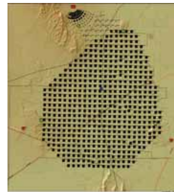
図1 TAの装置を四角形で示し、その北西部にあるTALEを丸で示す。黒は地表検出器を、赤は大気蛍光望遠鏡を示す。緑は通信塔を、青三角形は中央レーザー装置を示す。
