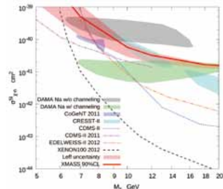
図3 スピンに依存しない場合のWIMP-核子の乱断面積の上限値曲線。バンドで示す領域は不定性によるもの。 Fig.3 Spin-independent elastic WIMP-nucleon cross section as a function of WIMP mass. The effect of uncertainty on the limit is shown in the band.
