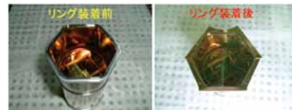
図5 バックグラウンド低減のために光電子増倍管に無酸素銅のリングを取り付けた所。 Fig.5 PMT with OFHC Copper ring to reduce the radioactive background
