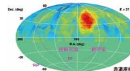
図5 TAで観測した10 19.76 電子ボルト以上の宇宙線の到来方向を20°でサンプリングした場合の統計的な有意度をプロットしたsky map (赤道座標表示)。赤経146.7°、赤緯43.2°を中心としたホットスポットが見られ、その最大有意度は5.1σである。
