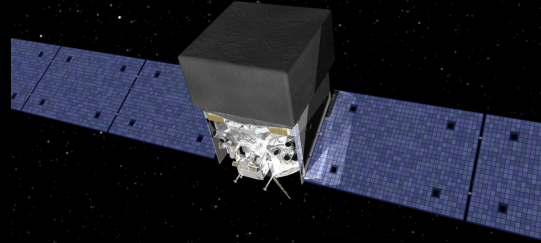
Fermi-LAT
