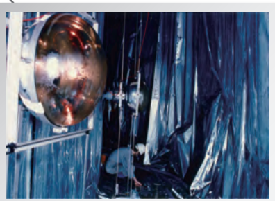
ノーベル賞受賞記念写真～その四： カミオカンデIIのための装置改造当時より
