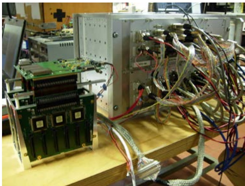
図 1: 調整中の焦点面検出器。ASIC ボード、1 次、2 次トリガボード、制御 CPU ボード、クロックボード等が接続されている。
