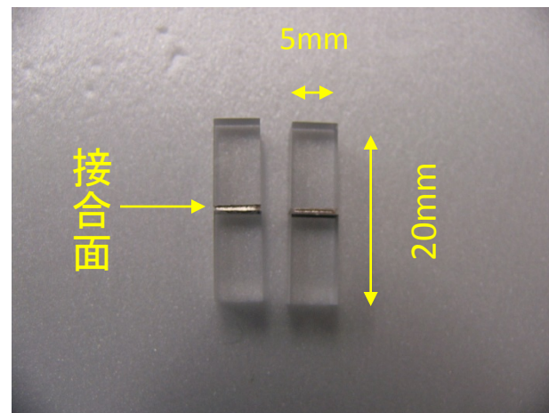
Mo-Mn法サファイア接合サンプル
