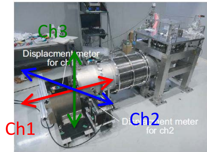
柏で実験中の冷凍機ユニット
