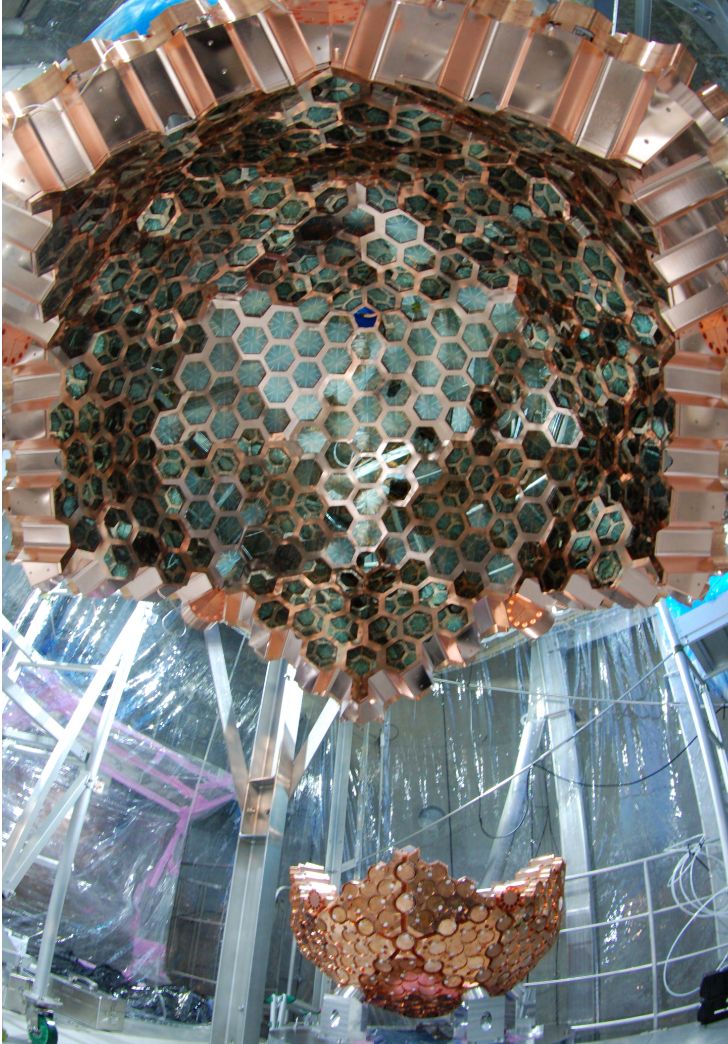
図1 光電子増倍管が並ぶ検出器の内部 (写真上) Inside of the XMASS Detector
