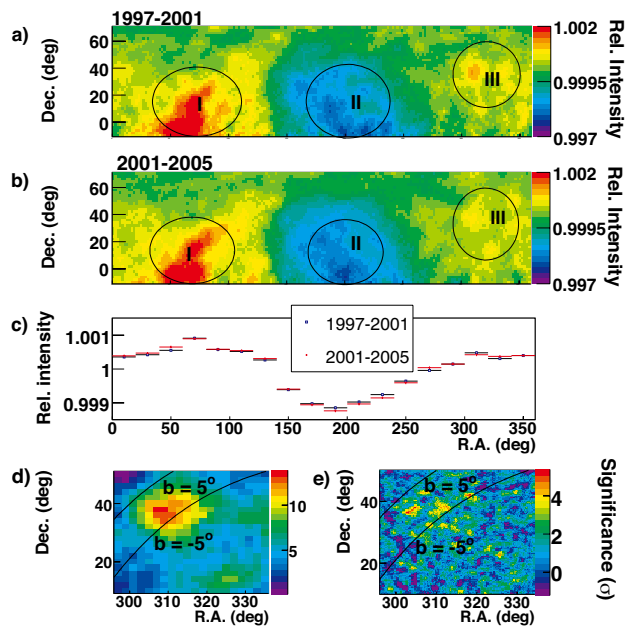
図6 シグナス領域 (III) のガンマ線点源探索 (e) の赤いホットスポットに注目) Search for gamma ray point sources in the Cygnus region (III). Watch out the hot red spots in e), please.
