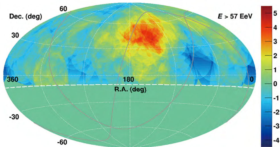
図5 TAで観測した 5.7 \times 10^{19} 電子ボルト以上の宇宙線の到来方向を半径 25° の円でオーバーサンプリングした場合の統計的有意性を示した天球マップ (赤道座標表示)。赤経 144.3°、赤緯 40.3° を中心としたところに赤く有意度の高いホットスポットが見られる。 Hammer projection of the statistical significance of TA cosmic ray events with energies greater than 5.7 \times 10^{19} eV with 25°-radius circle oversampling in the equatorial coordinates. The maximum excess appears as a hotspot centered at right ascension of 144.3° and declination of 40.3°.
