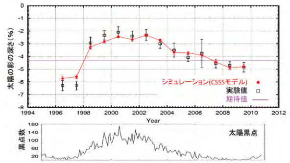
図4 観測された宇宙線中の太陽の影の深さに関するデータシミュレーションの比較⊕と、太陽黒点数の年変化⊕ Comparison of Sun shadow depth in cosmic rays between MC and simulation and the observed data. (Top) Yearly variation of sun spot numbers. (Bottom)
