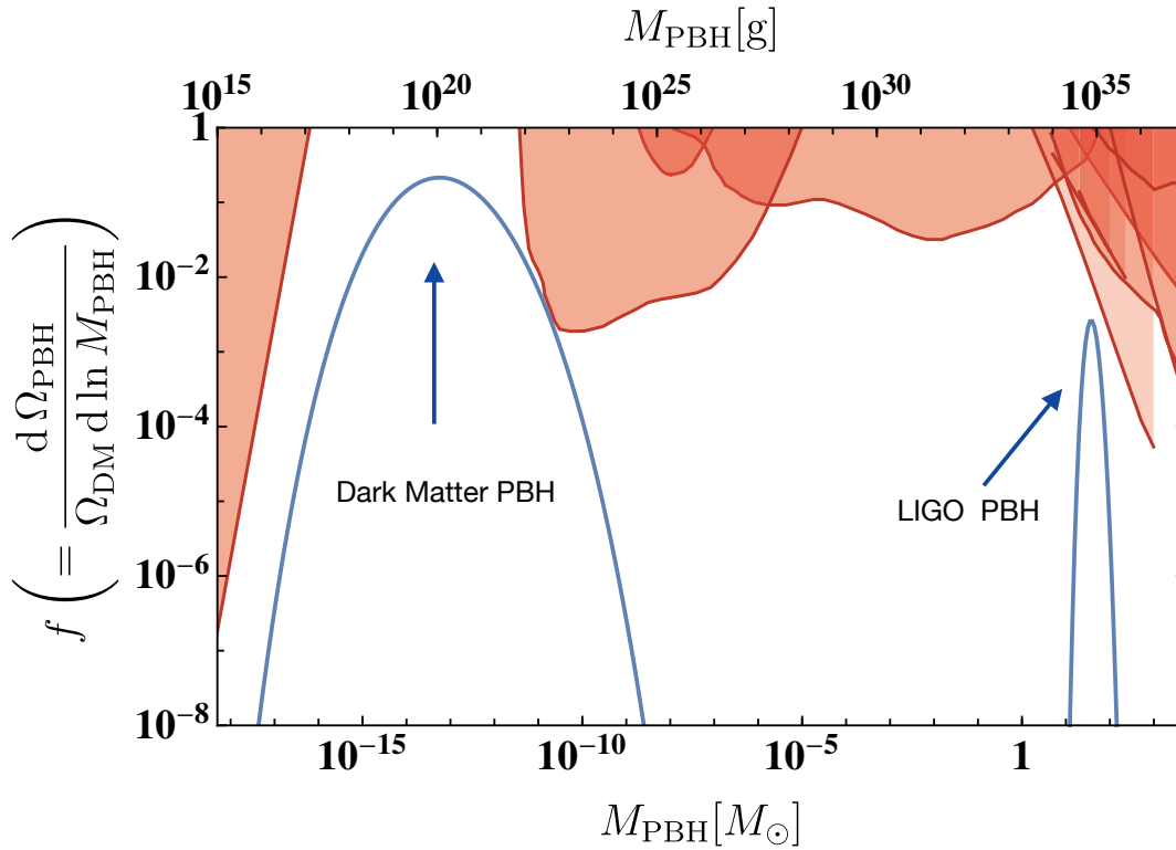
図1 ダブル・インフレーションで生成される原始ブラックホール (PBH) の質量分布。実線が理論的の予言を表し、オレンジの領域が観測の制限を表す。質量の軽い PBH は宇宙の暗黒物質を説明し、質量が大きな PBH は重力波検出器 LIGO で見つかったイベントを説明できる。 Mass distribution of primordial black holes (PBHs). Solid curves represent the theoretical prediction and the orange shadows show the present observational constraints. Light PBHs can account for dark matter of the universe and heavy PBHs can explain the gravitational wave events discovered by LIGO.
