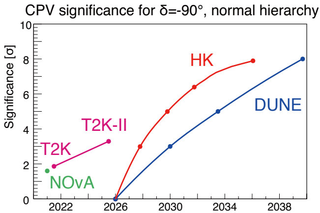
図3 CPの破れの発見能力(有意度)をハイパーカミオカンデ(HK)と米国計画(DUNE)、現行実験(T2K、NOvA)と比較したものの。横軸は年。 Expected significance of CP violation observation for Hyper-Kamiokande (HK), US-based project (DUNE), running experiments (T2K, NOvA). X-axis is year.
