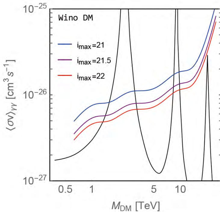
図2 ガンマ線に対消滅するウィーノ型暗黒物質に対する CTA 実験で期待される感度曲線。ここでは矮小楕円体銀河 Ursa Major II, Coma Berenices, Seque 1, Ursa Major I を 50 時間ずつ測定することを仮定。(黒：理論計算による対消滅断面積。青、紫、赤：矮小楕円体銀河からのガンマ線に対する CTA 実験感度。i_max は暗黒物質密度測定に用いる矮小銀河星の上限等級) Sensitivity lines of CTA for Wino dark matter annihilating into two photons. Here, we assume 50 hours observation for the ultra-faint dwarf spheroidal galaxies, Ursa Major II, Coma Berenices, Seque 1, and Ursa Major I. (Black line: the predicted annihilation cross section. Colored lines : The sensitivity lines of CTA for given upper bounds on the member star magnitude used to estimate the dark matter density in the dwarf spheroidal galaxies.)
