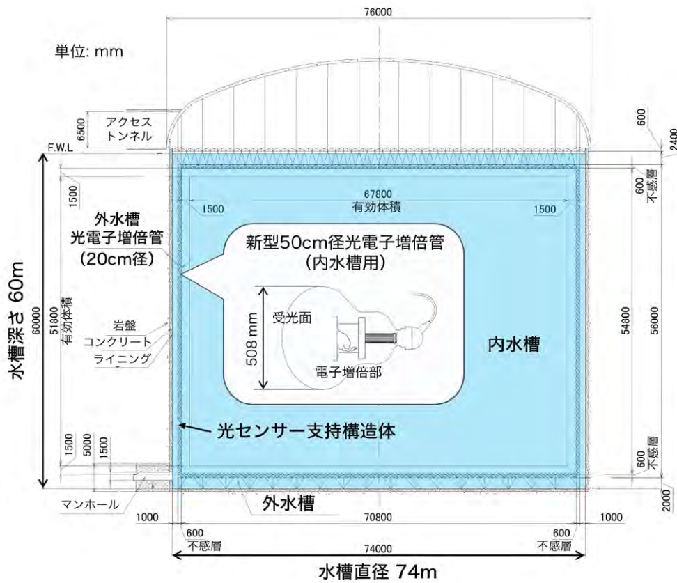
図1 ハイパーカミオカンデ装置の概念図 Schematic view of the Hyper-Kamiokande
