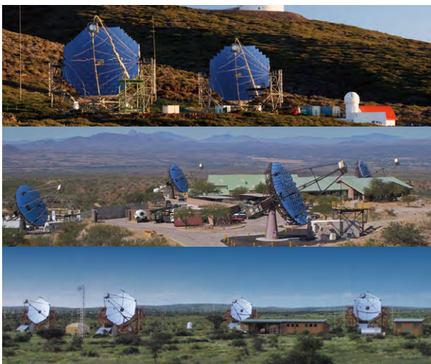
図 1 現在稼働中の超高エネルギーガンマ線望遠鏡。写真上から MAGIC, VERITAS, H.E.S.S. The current generation VHE gamma ray observatories, the MAGIC, VERITAS, and H.E.S.S. telescopes
