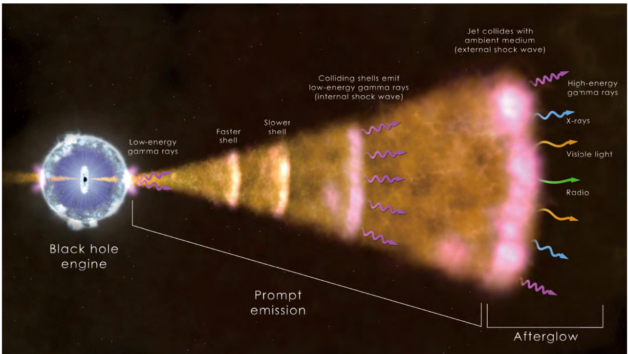
図2 ガンマ線バーストの想像図。巨星がその寿命に至り、中心核が重力崩壊を起こし、ブラックホールを形成する。そこへ星のガスが降着し、細く絞られた相対論的なジェットを放つ。ジェットは星表面を突き破り、星間空間へ飛び出す。そこで衝撃波を形成し、数十秒間に渡ってガンマ線を放ったり、徐々に暗くなる電波からX線での残光を放ったりする。©NASA's Goddard Space Flight Center Description of gamma-ray burst. When the collapse of a very massive star at the end of its life forms a black hole. Gas in the star accretes onto the black hole. Then, the black hole produces well-collimated relativistic jets. The jets break out the surface of the star, and propagate in the interstellar space. Shocks formed in the jets or interstellar medium are considered to be responsible for the prompt gamma-ray emission and the afterglow emission, respectively.
