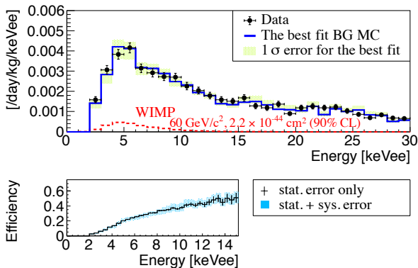
図5 実際に観測されたデータ (黒点) とノイズ事象の予測分布 (青線)。赤い点線はノイズに埋もれている可能性のある WIMPs 信号の上限值。 The energy spectrum of data after the selection of events (black) and the best fit of background model (blue) are shown together with a 2.2 \times 10^{-44} cm 2 cross section at the 90% CL (red).
