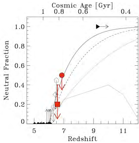
図5 これまでの研究で明らかにされた宇宙再電離の歴史。赤方偏移（横軸）に対する中性水素比（縦軸）の進化。赤印が Suprime-Cam の探査から付けられた制限。4つの曲線は異なる理論モデル。いつ、どのように宇宙再電離が進んできたかはほとんど分かっていない。 History of cosmic reionization, so far, understood. Red symbols denote constraints from our Suprime-Cam survey. Four lines represent different theoretical predictions. The epoch and process of cosmic reionization are unknown.
