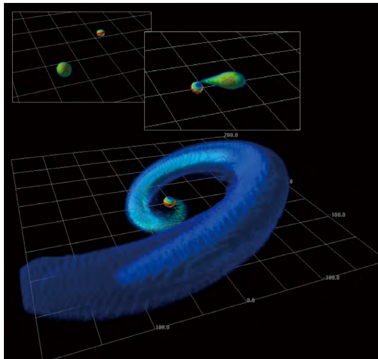
図3 ブラックホールと中性子星の連星合体シミュレーションの例。重力波を放出し軌道エネルギーを失い次第に連星間距離を縮め、やがて合体する。合体時には一部の物質がブラックホール降着円盤を形成し、さらに一部が系外に放出される。ブラックホール降着円盤や放出物質は突発的電磁波現象の源となるため、こうした重力波と電磁波を予測する事で観測から連星合体の物理に迫る事が出来る。 Numerical simulation for a black-hole neutron star merger. The orbital separation shrinks gradually via the gravitational-radiation reaction, and eventually the two objects merge. A black-hole accretion disk is formed and a fraction of neutron-star material is ejected from the system after the merger. These black-hole accretion disk and ejected material will be the sources of transient electromagnetic phenomenon. Simultaneous detection of gravitational and electromagnetic waves from binary mergers enables us to study physics in the extreme environment.
