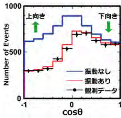
図2 大気ニュートリノの天頂角分布。上向きニュートリノの振動の証拠 Zenith-angle distribution of atmospheric neutrinos, showing evidence of oscillation for upward-going neutrinos
