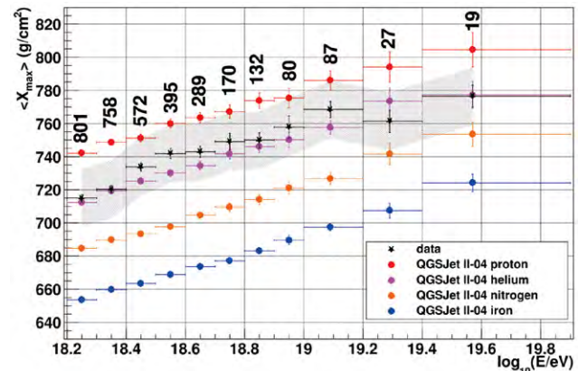
図4 TAで測定した超高エネルギー宇宙線の平均 Xmax とエネルギーの関係 (●)。赤、紫、橙、青色の丸印がそれぞれ陽子、ヘリウム、窒素、鉄モデルである。 The average Xmax vs. energy of TA cosmic ray events (●). The red, purple, orange and blue circles denote proton, helium, nitrogen and iron models, respectively.
