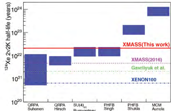
図4 124 Xe の 2 ニュートリノ二重電子捕獲事象の半減期と、いくつかの理論的予測値との比較。実験的な下限値が、いくつかの理論モデルの予測する領域を排除していることが分かる。 Comparison of the experimental limit on 124 Xe two-neutrino double-electron-capture half-life with some theoretical predictions. The experimental result excluded some of the theoretical calculations.
