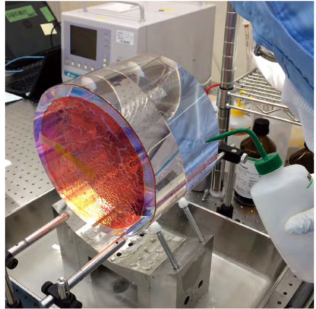
図4 直径 22 cm の無色透明のサファイアの鏡 A transparent sapphire mirror 22 cm in diameter
