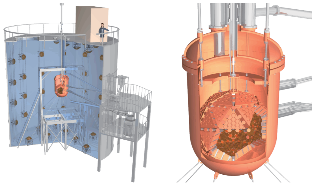
2 液体キセノン検出器 ⑥、と水放射線シールドの概念図 The schematic view of the detector and the water tank
