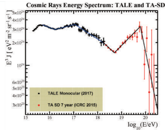
3 TAの地表検出器(●)とTALE望遠鏡(●)で測定した超高エネルギー宇宙線のエネルギースペクトル。 Energy spectra of UHECRs measured with the TA surface detector (●) and the TALE telescope (●).
