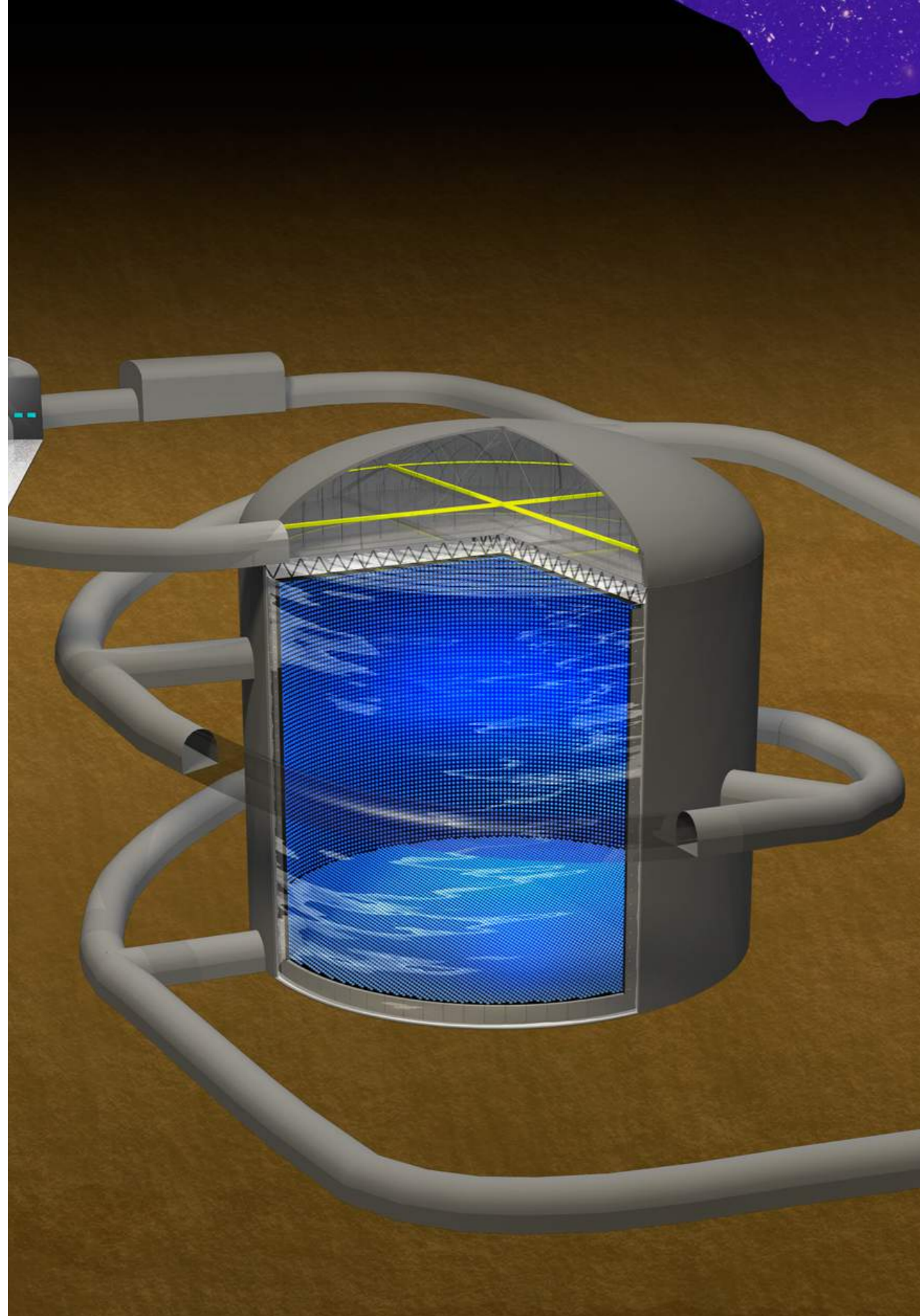
Hyper-Kamiokande
