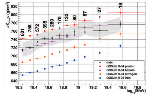
4 TAで測定した超高エネルギー宇宙線の平均Xmaxとエネルギーの関係(●)。赤、紫、橙、青色の丸印がそれぞれ陽子、ヘリウム、窒素、鉄モデルである。 The average Xmax vs. energy of TA cosmic ray events (●). The red, purple, orange and blue circles denote proton, helium, nitrogen and iron models, respectively.
