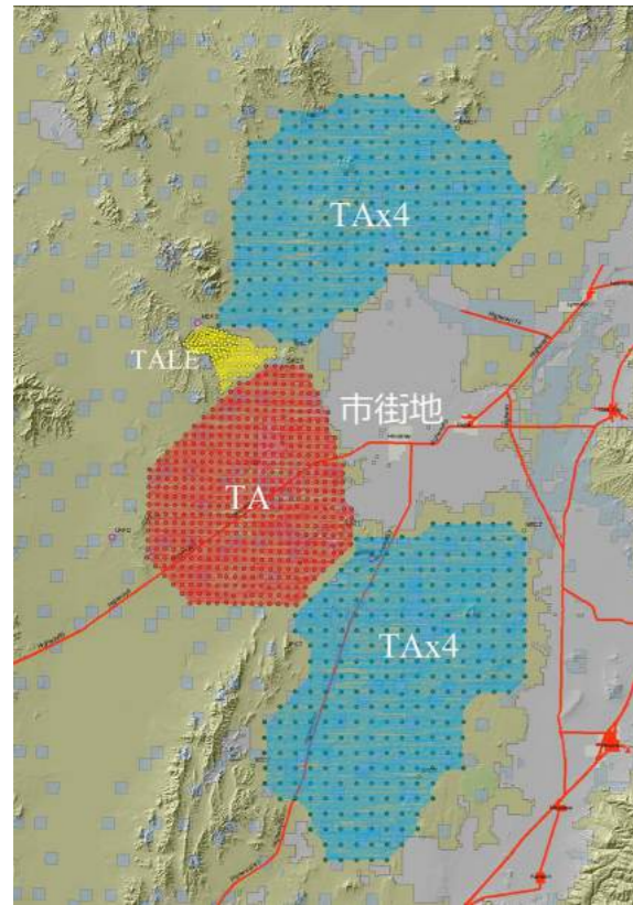
2 テレスコプアレイ(TA)とTAx4、TALEの検出器の設置範囲。 Arrangement area of the detector of TA, TA×4 and TALE experiment
