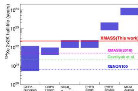
5 124 Xe の 2 ニュートリノ二重電子捕獲事象の半減期と、いくつかの理論的予測値との比較。実験的な下限値が、いくつかの理論モデルの予測する領域を排除していることが分かる。 Comparison of the experimental limit on 124 Xe two-neutrino double-electron-capture half-life with some theoretical predictions. The experimental result excluded some of the theoretical calculations.
