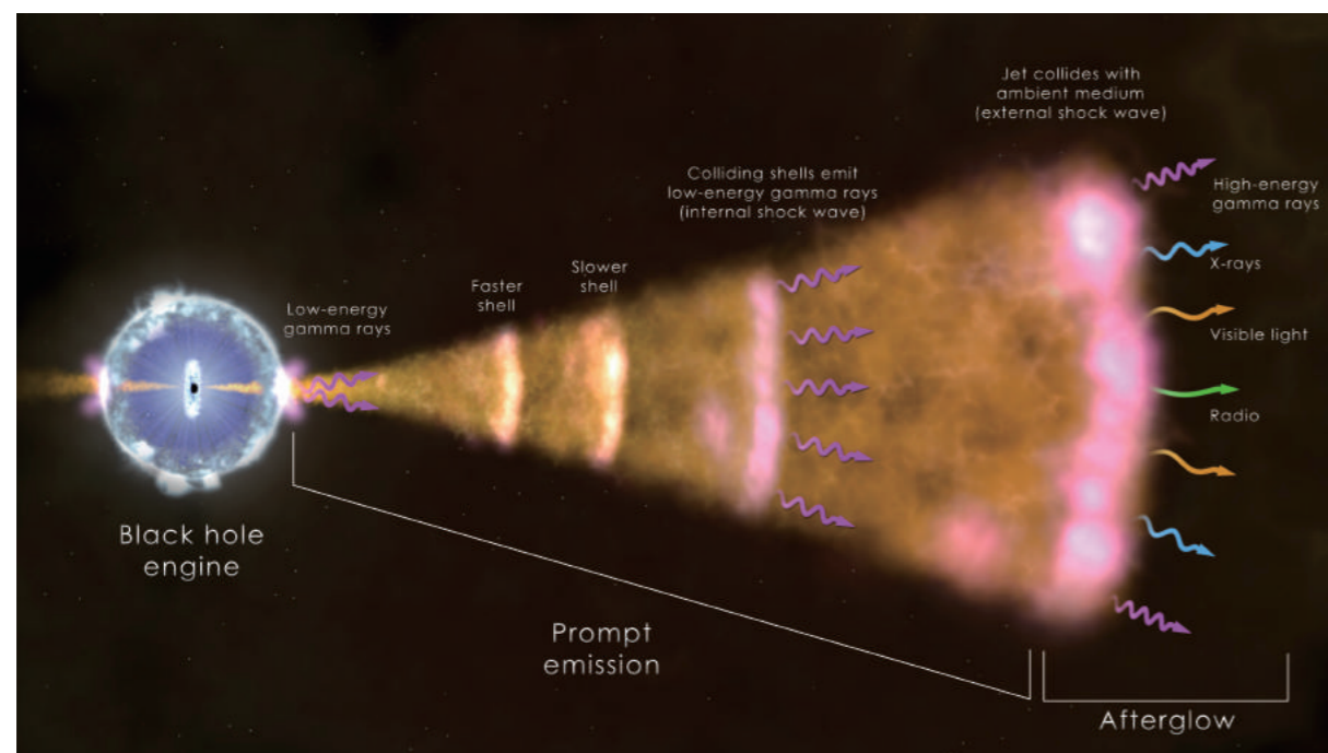
2 ガンマ線バーストの想像図。巨星がその寿命に至り、中心核が重力崩壊を起こし、ブラックホールを形成する。そこへ星のガスが降着し、細く絞られた相対論的なジェットを放つ。ジェットは星表面を突き破り、星間空間へ飛び出す。そこで衝撃波を形成し、数十秒間に渡ってガンマ線を放ったり、徐々に暗くなる電波からX線の残光を放ったりする。©NASA's Goddard Space Flight Center
