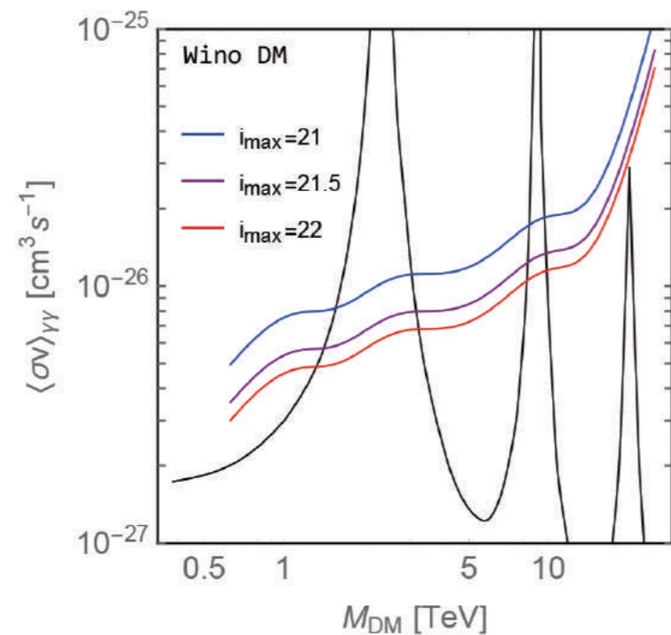
2 ガンマ線に対消滅するウィーノ型暗黒物質に対する CTA 実験で期待される感度曲線。ここでは矮小楕円体銀河 Ursa Major II, Coma Berenices, Seque 1, Ursa Major I を 50 時間ずつ測定することを仮定。(黒: 理論計算による対消滅断面積。青、紫、赤: 矮小楕円体銀河からのガンマ線に対する CTA 実験感度。imax は暗黒物質密度測定に用いる矮小銀河星の上限等級)
