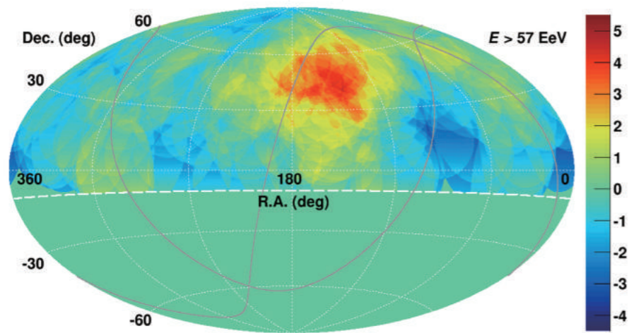
5 TAで観測した 5.7 \times 10^{19} 電子ボルト以上の宇宙線の到来方向を半径 25^\circ の円でオーバーサンプリングした場合の統計的な有意度を示した天球マップ(赤道座標表示)。赤経 144.3^\circ 、赤緯 40.3^\circ を中心としたところに赤く有意度の高いホットスポットが見られる。 Hammer projection of the statistical significance of TA cosmic ray events with energies greater than 5.7 \times 10^{19} eV with 25^\circ -radius circle oversampling in the equatorial coordinates. The maximum excess appears as a hotspot centered at right ascension of 144.3^\circ and declination of
