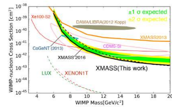
3 季節変動によるスピンの依存しない場合の WIMP-核子の散乱断面積の上限値曲線。季節変動解析によって DAMA/LIBRA 領域を殆ど排除した Upper limit on the spin-independent elastic WIMP-nucleon cross section as a function of WIMP mass by an annual modulation analysis. XMASS excluded the most of the allowed region of DAMA/LIBRA experiment
