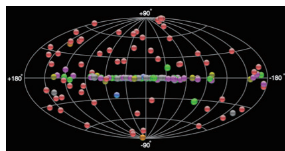
2 超高エネルギーガンマ線源 (>100GeV) を銀河座標系に示したものである。200 に近い銀河内、銀河系外のガンマ線源が発見されている。Very High Energy Gamma Ray Sky (>100GeV). About 200 Galactic and extragalactic sources have been discovered.
