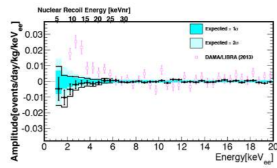
4 ダークマターモデルに依存しない探索。季節変動を用いて得られた振幅とエネルギーの関係を示す。XMASS 実験では有意な振幅は得られず、DAMA/LIBRA 実験の結果を再現しなかった Model independent analysis by an annual modulation search. XMASS obtained strong upper limits on the amplitude in the low energy regions and could not reproduce the DAMA/LIBRA result.
