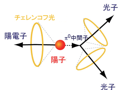
4 陽子が陽電子とπ⁰中間子に崩壊する様子 A proton decays to a positron and a neutron pion
