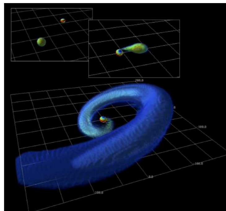
3 ブラックホールと中性子星の連星合体シミュレーションの例。重力波を放出し軌道エネルギーを失い次第に連星間距離を縮め、やがて合体する。合体時には一部の物質がブラックホール降着円盤を形成し、さらに一部が系外に放出される。ブラックホール降着円盤や放出物質は突発的電磁波現象の源となるため、こうした重力波と電磁波を予測する事で観測から連星合体の物理に迫る事が出来る。
