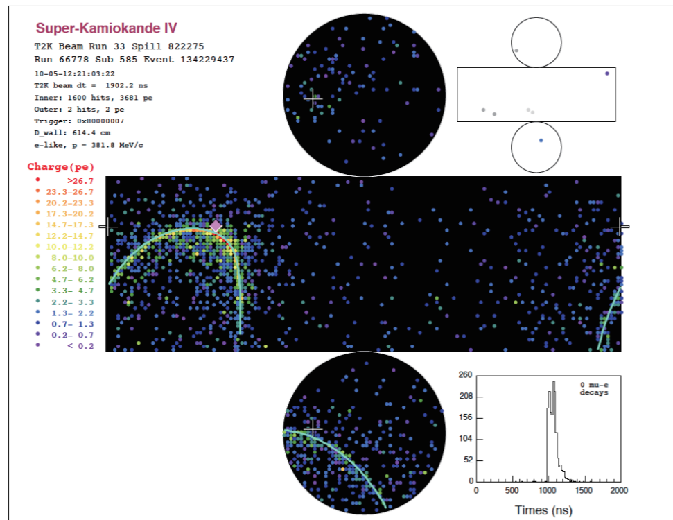
1 スーパーカミオカンデで観測された、電子ニュートリノ反応候補事象の一つ。円筒形をしたスーパーカミオカンデの展開図で、内壁に配置された光電子増倍管の内、光を捉えたものにとらえた光の強度に応じて色をつけて表示している。水と電子型ニュートリノ反応によって発生した電子が引き起こす電子・陽電子シャワーが発したチェレンコフ光がリング状に捉えられている。
