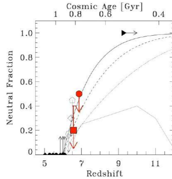
5 これまでの研究で明らかにされた宇宙再電離の歴史。赤方偏移 (横軸) に対する中性水素比 (縦軸) の進化。赤印が Suprime-Cam の探査から付けられた制限。4つの曲線は異なる理論モデル。いつ、どのように宇宙再電離が進んできたかはほとんど分かっていない。 History of cosmic reionization, so far, understood. Red symbols denote constraints from our Suprime-Cam survey. Four lines represent different theoretical predictions. The epoch and process of cosmic reionization are unknown.
