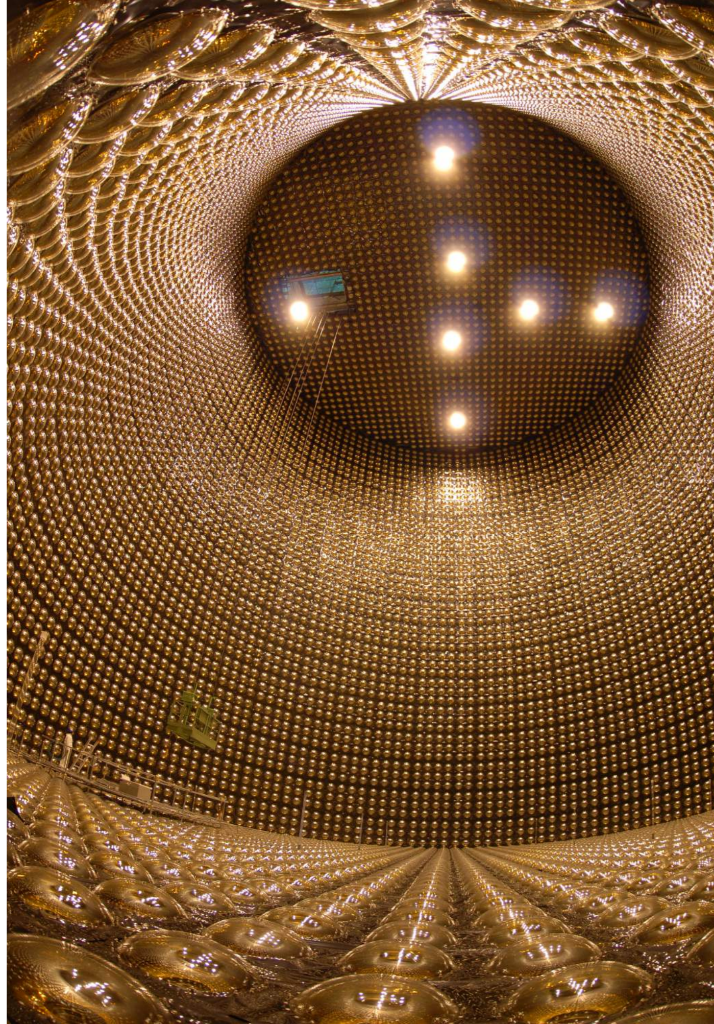
Super-Kamiokande
