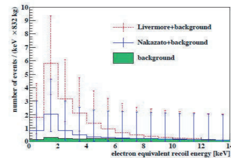
6 銀河の中心での超新星爆発を XMASS で観測した場合のニュートリノスペクトル(シミュレーション)。バックグラウンド(緑)は小さく無視でき、ニュートリノ事象が確実に捉えられることが分かる。 Neutrino spectrum in XMASS (Simulation data). The supernova at the Galactic center is assumed. Comparing the background (Green), it is clearly shown that the supernova neutrinos can be detected with XMASS.
