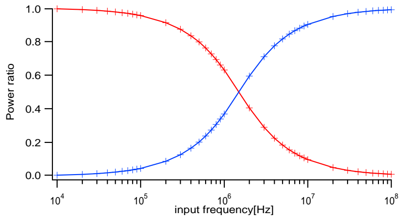
図 3: フィルタのローパス側、ハイパス側の消費電力比
