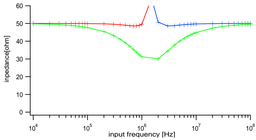
図 2: フィルタのトータルのインピーダンス
