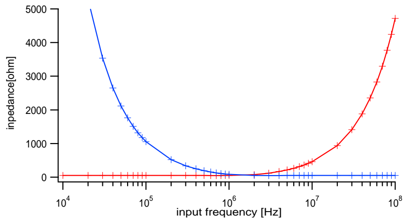
図 1: フィルタのローパス側、ハイパス側のインピーダンス
